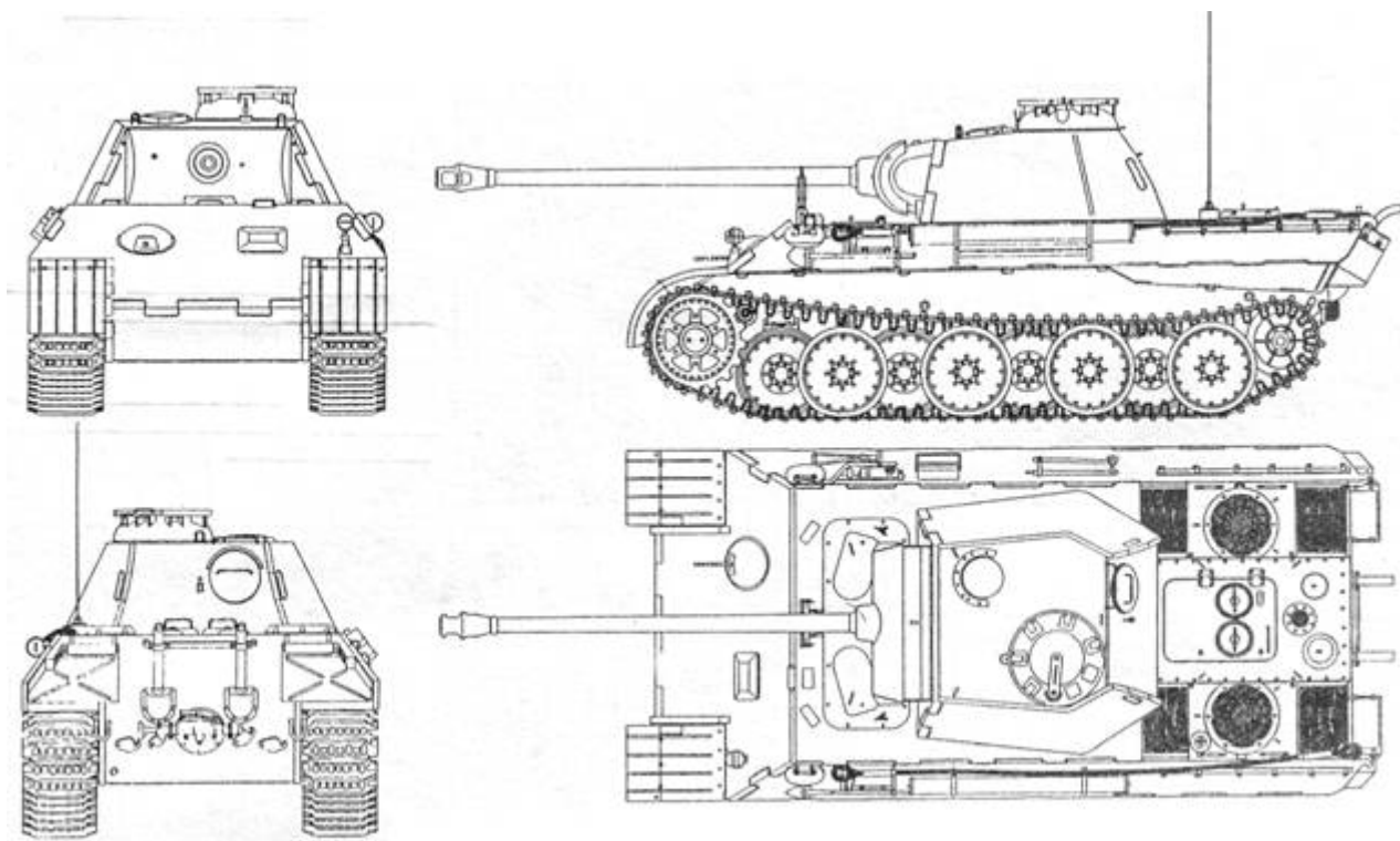
Танк "Пантера"
